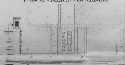
Coupe de l'entrée de l'air extérieur
