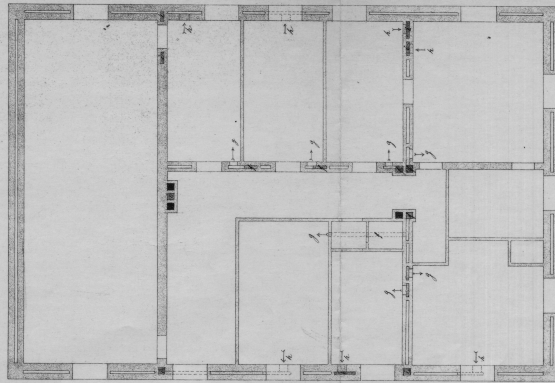
Plan du premier Etage
